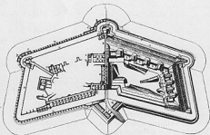
256. Detachiertes Fort. Aus Meyers Konversationslexikon.
